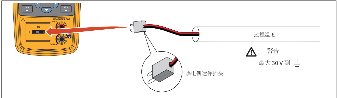
图 7. 使用热电偶测量温度
