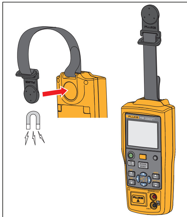
图 5. 使用本产品的磁性挂带
