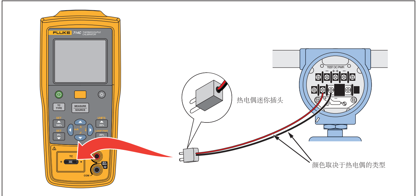
图 8. 用于模拟热电偶的连接
