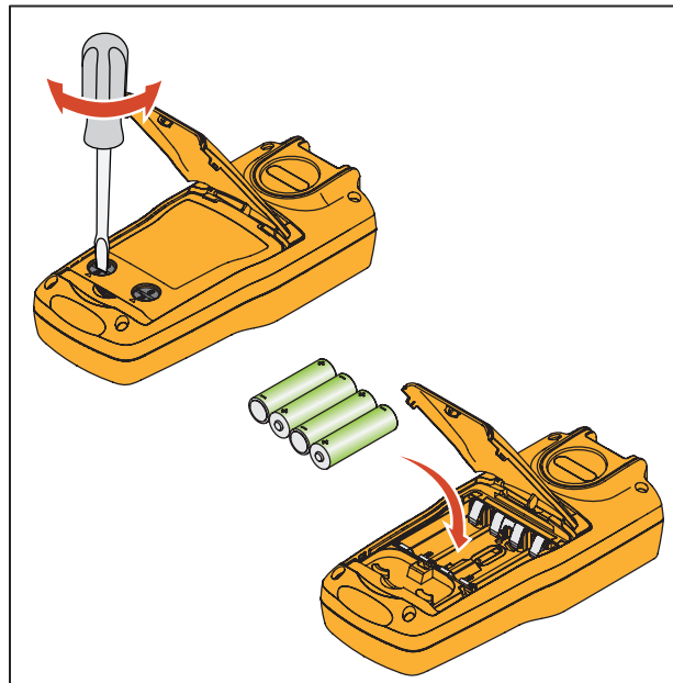
图 9. 更换电池
