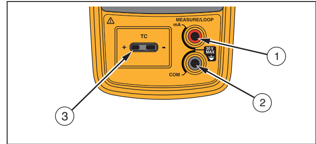
图 2. 输入/输出端子和连接器
