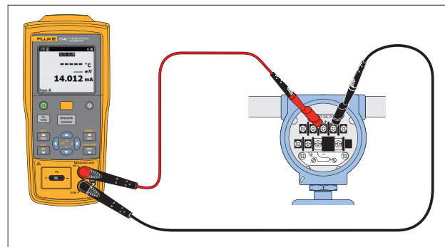
图 6. 激活回路电源的连接
